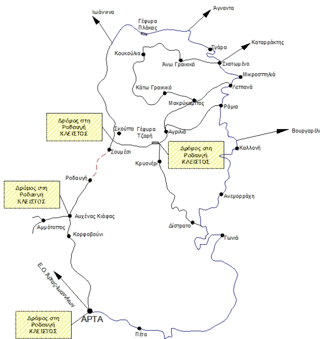
ΣΧΕΔΙΑΓΡΑΜΜΑ ΡΥΘΜΙΣΗΣ ΚΥΚΛΟΦΟΡΙΑΣ ΚΑΤΑ ΤΗ ΔΙΑΡΚΕΙΑ ΤΩΝ ΕΡΓΑΣΙΩΝ ΑΠΟΚΑΤΑΣΤΑΣΗΣ ΤΟΥ ΟΔΟΣΤΡΩΜΑΤΟΣ ΣΤΗ ΡΟΔΑΥΓΗ (από 04.03.2013 - 04.04.2013)
